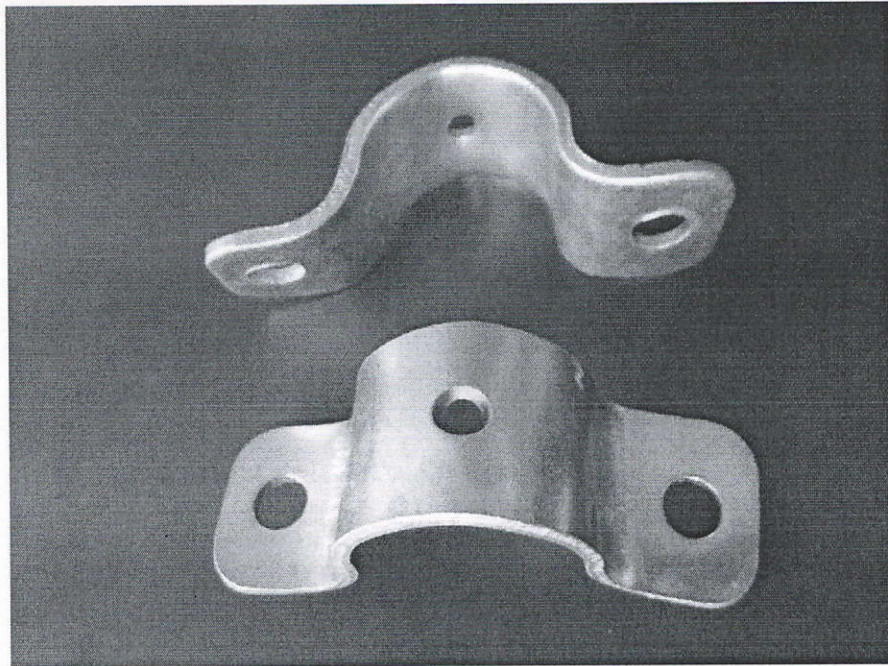
Рисунок А.1 – Внешний вид хомутов
